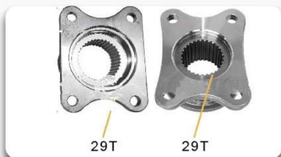
Yoke
